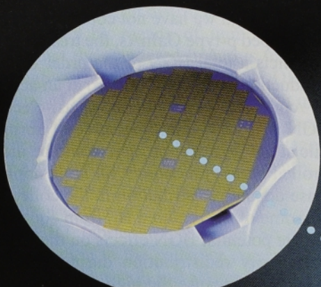
TMGa
