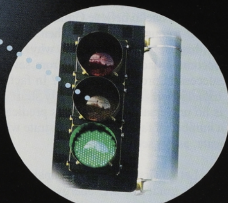
CP 2 Mg
